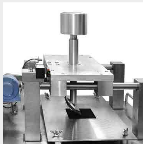
Přístroj na provádění podpatkového testu
