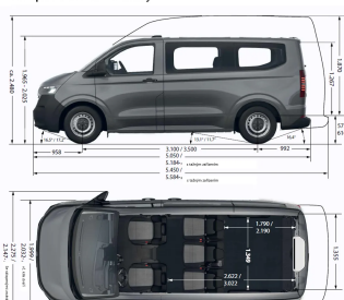
transporter kombi - rozměry
