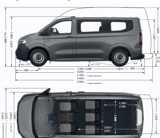
transporter kombi - rozměry
