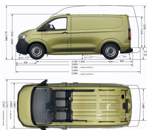
Transporter skříňový - rozměry
